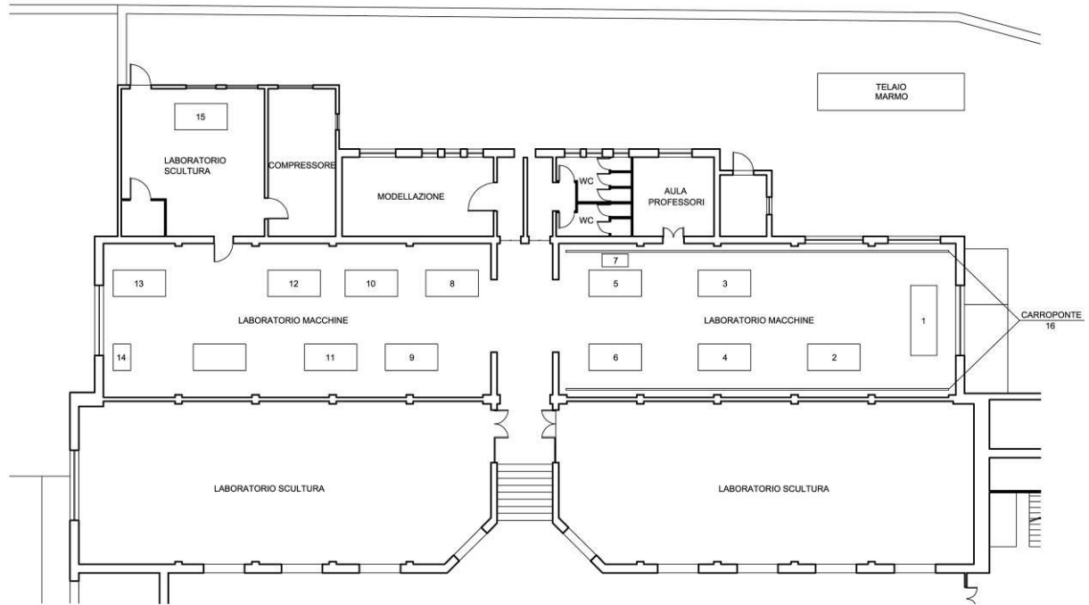
PIANTA LABORATORI PIANO TERRA
